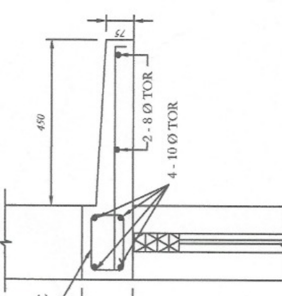
DET. OF R.C.C. LINTEL & CHAJJA SCALE: 1:10
